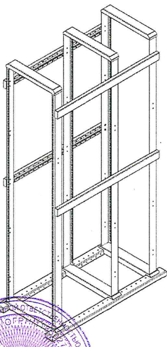
Стойка телекоммуникационная универсальная трехрамная
